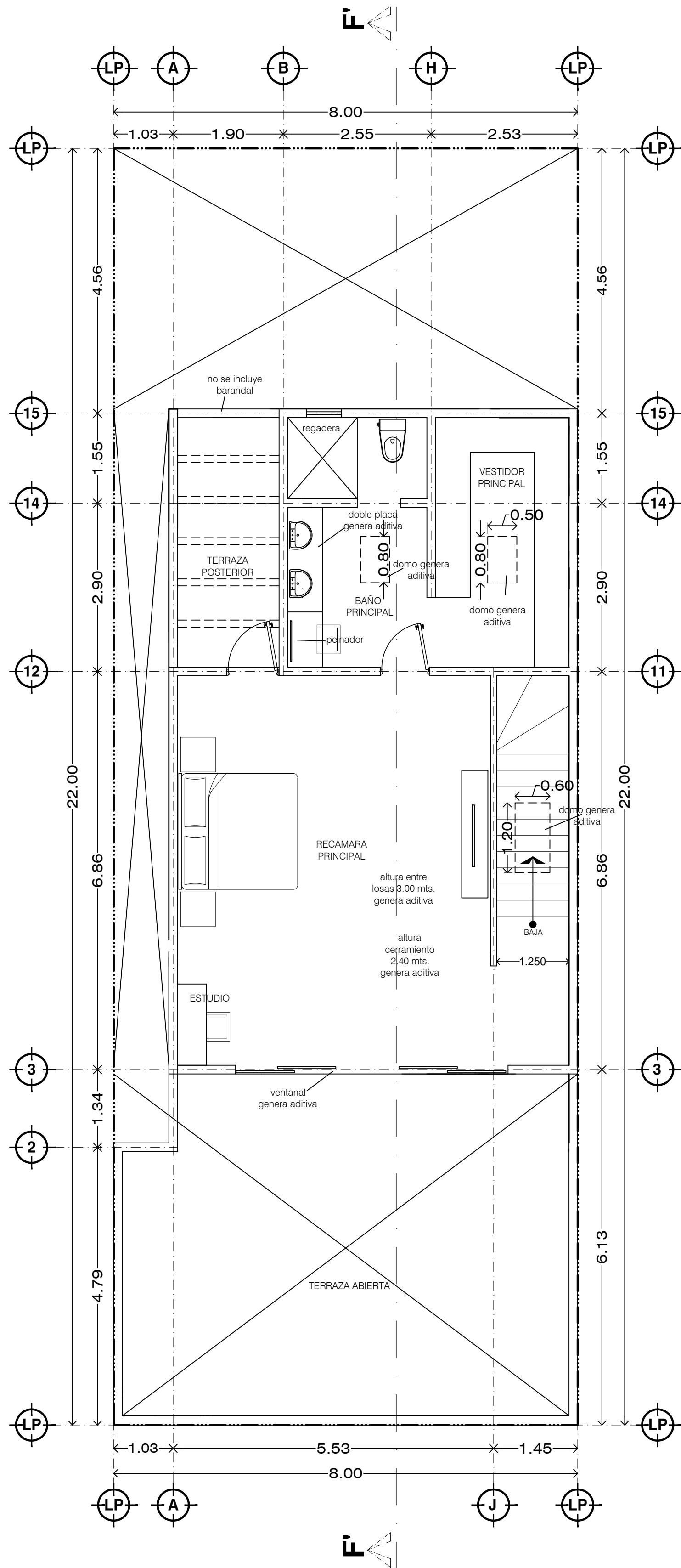
72.34 m2 PLANTA TERRAZA
