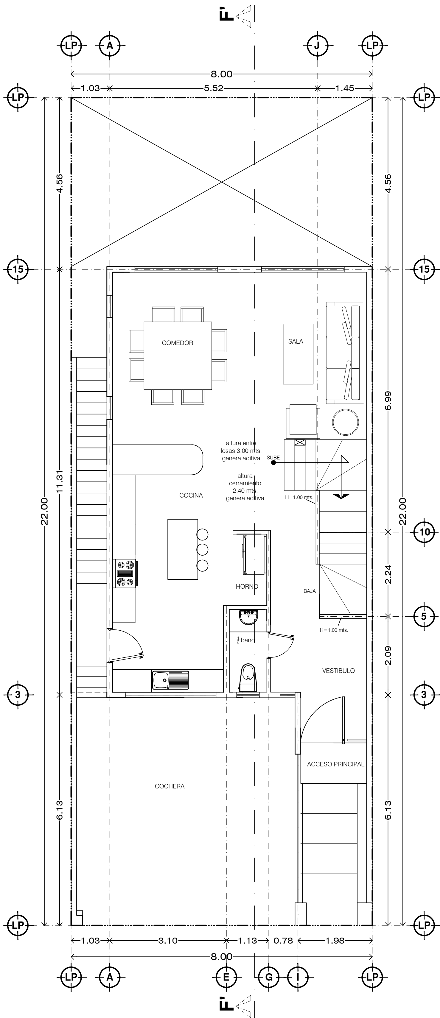
129.34 m2 PLANTA BAJA
