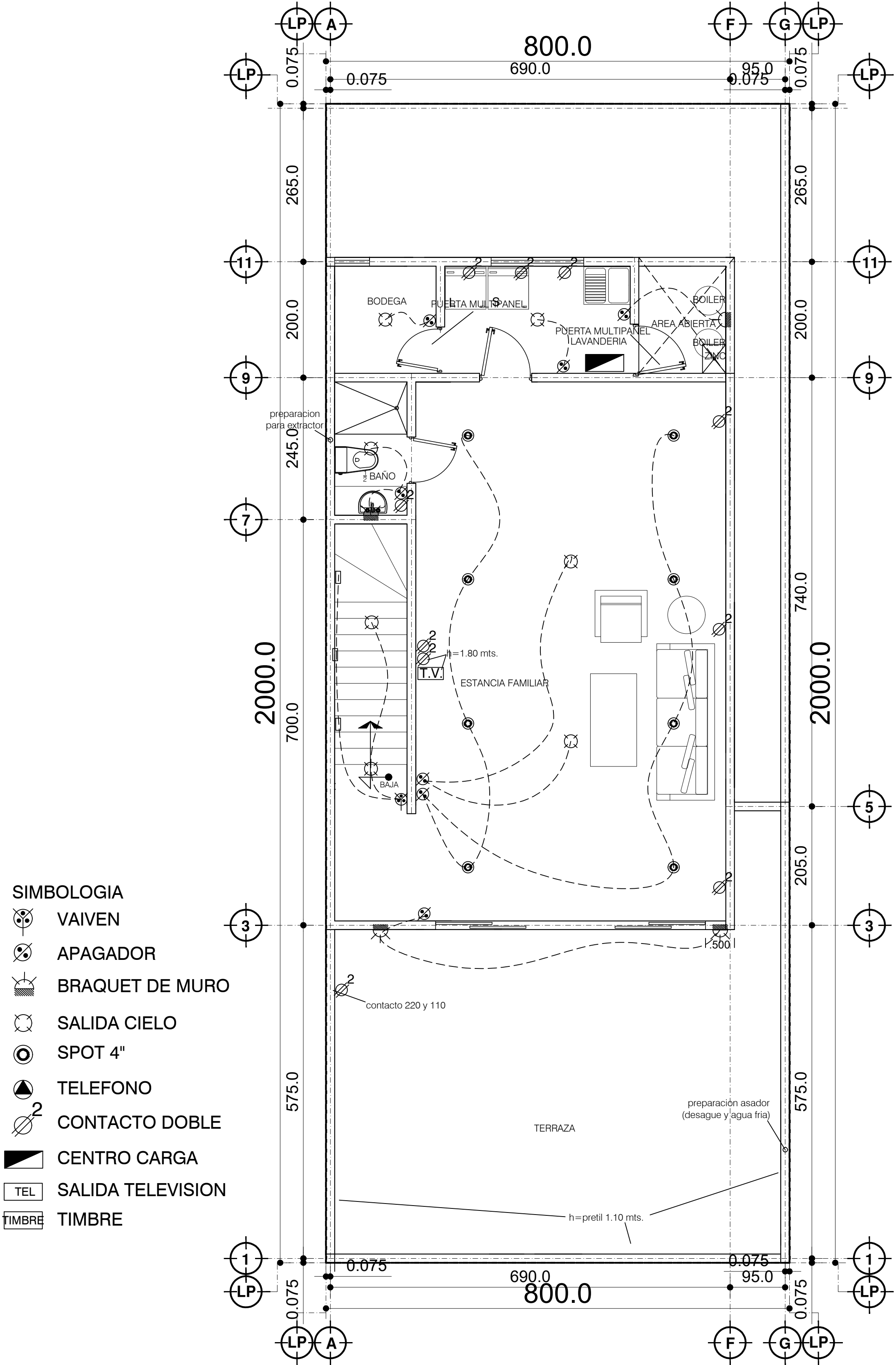
PLANTA TERRAZA PLANO ELECTRICO
