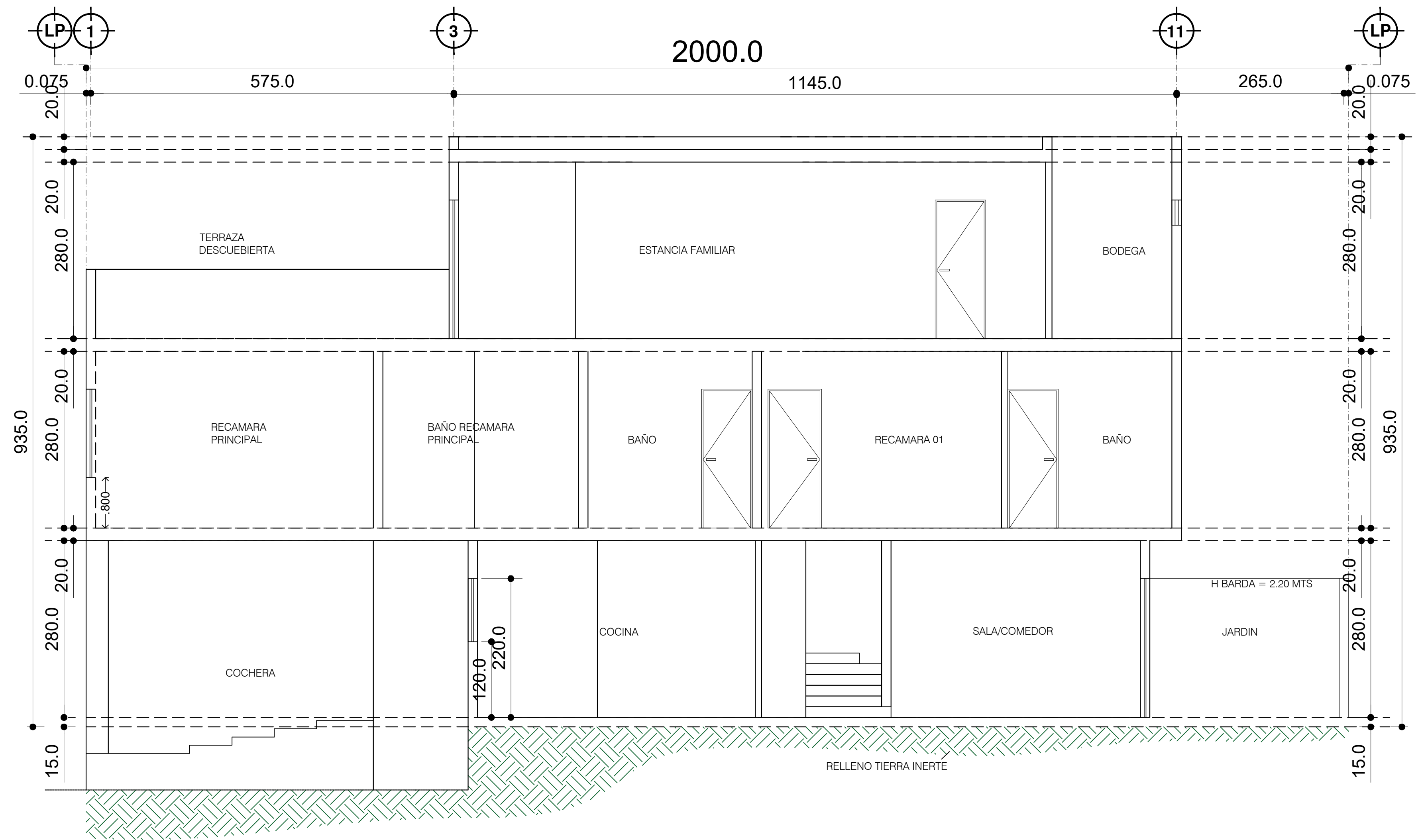
CORTE LONGITUDINAL 1-1'
