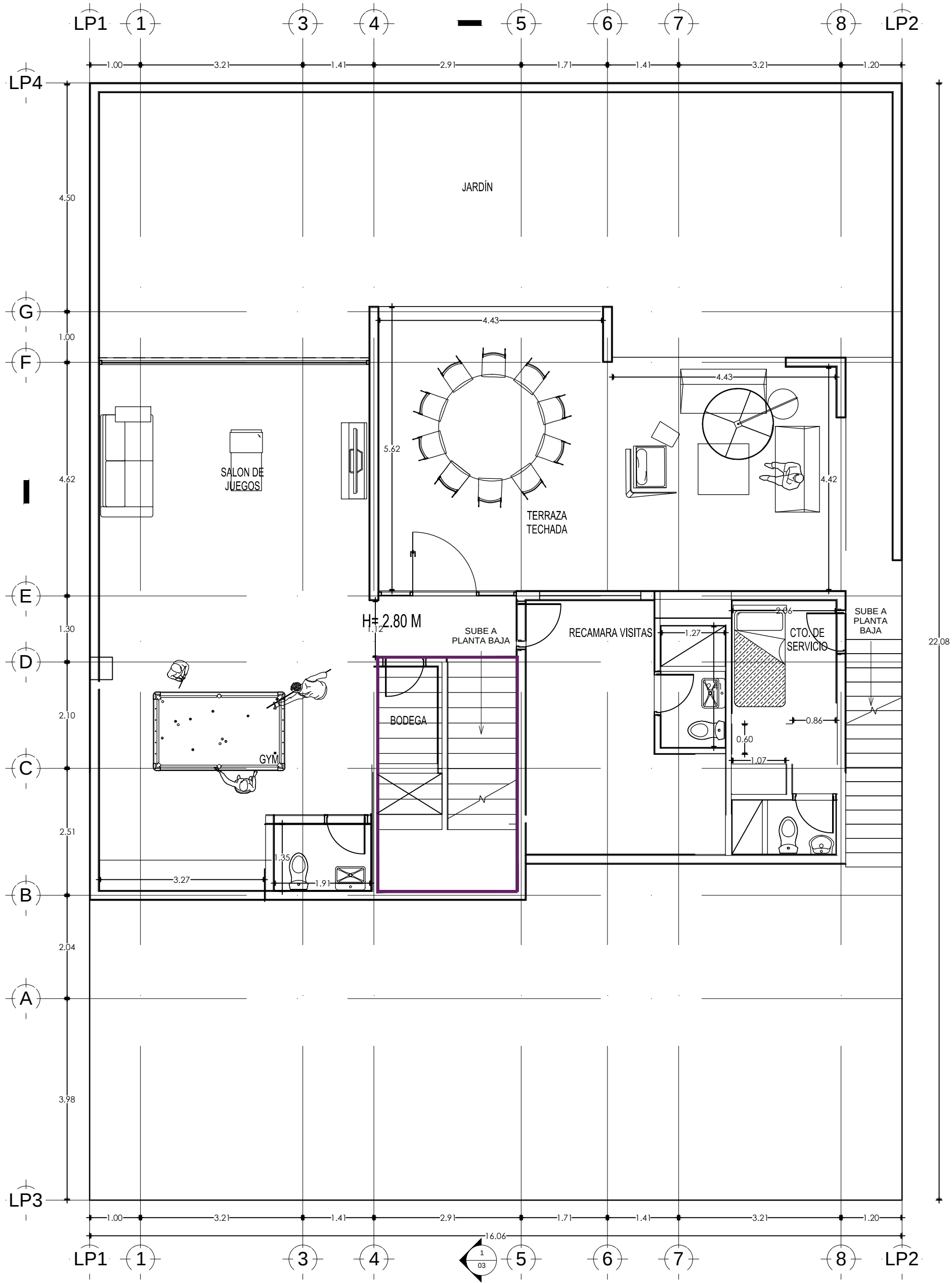
PLANTA SOTANO 160.50 m2 SR. DANIEL PALACIOS
