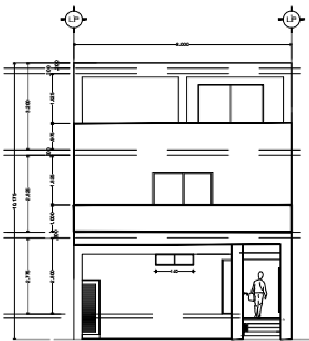
FACHADA VISTA FRONTAL
