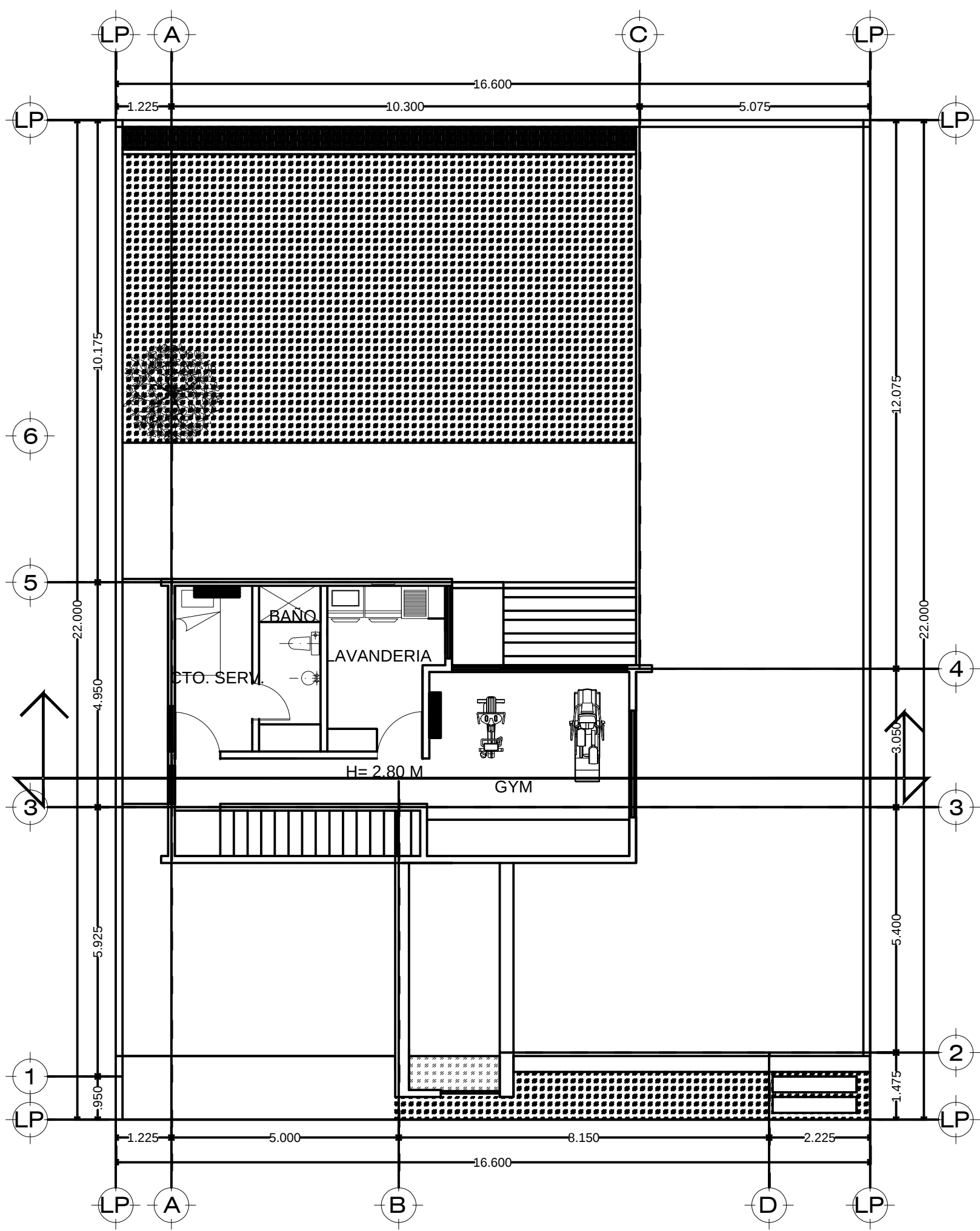
PLANTA TERRAZA 56.58
