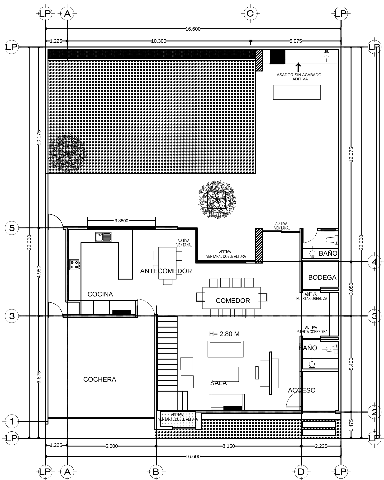
PLANTA BAJA 218.49
