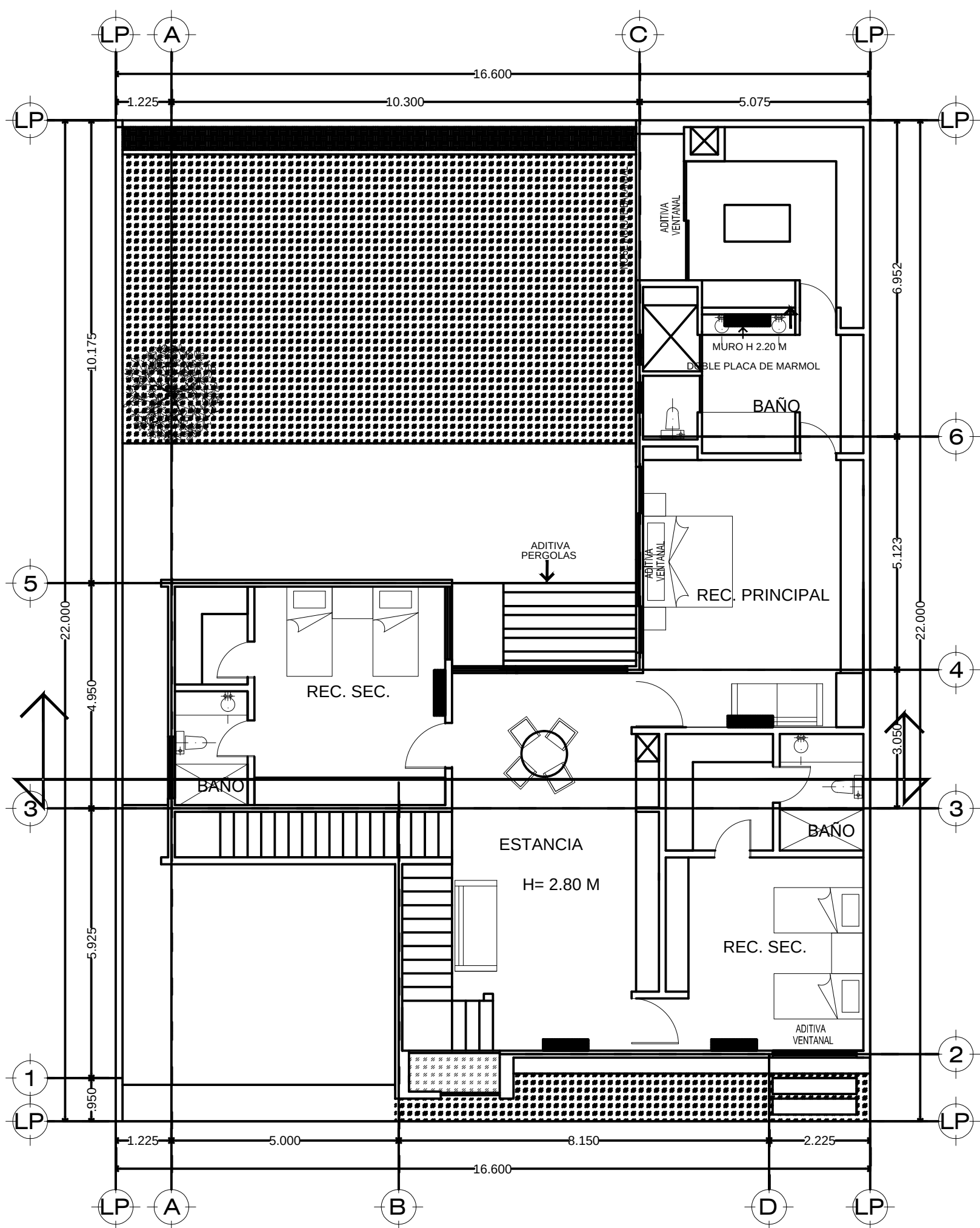
PLANTA ALTA 185.29
