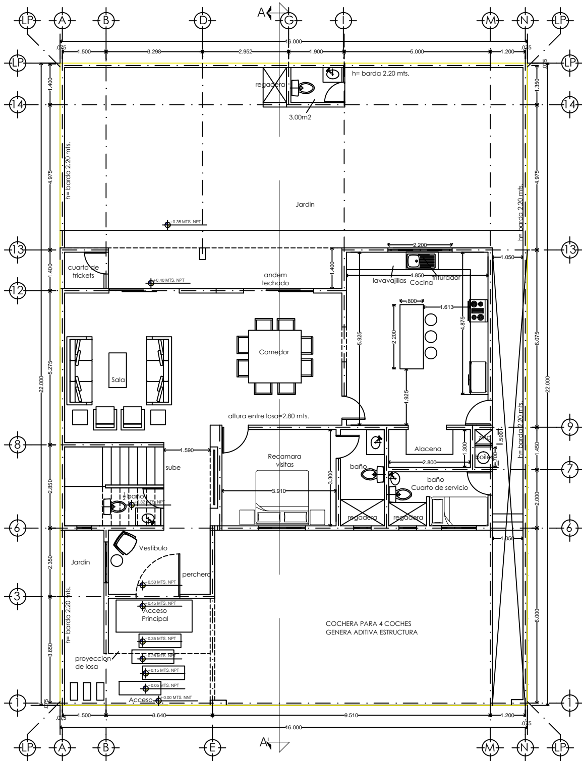
Planta baja 219.26 m 2
