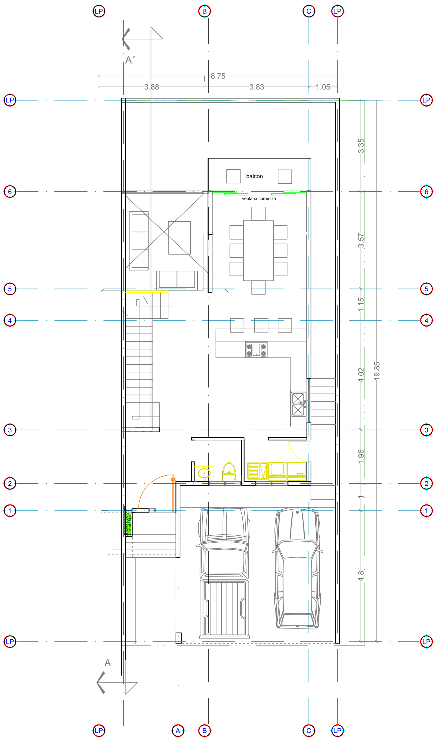
PLANTA BAJA
