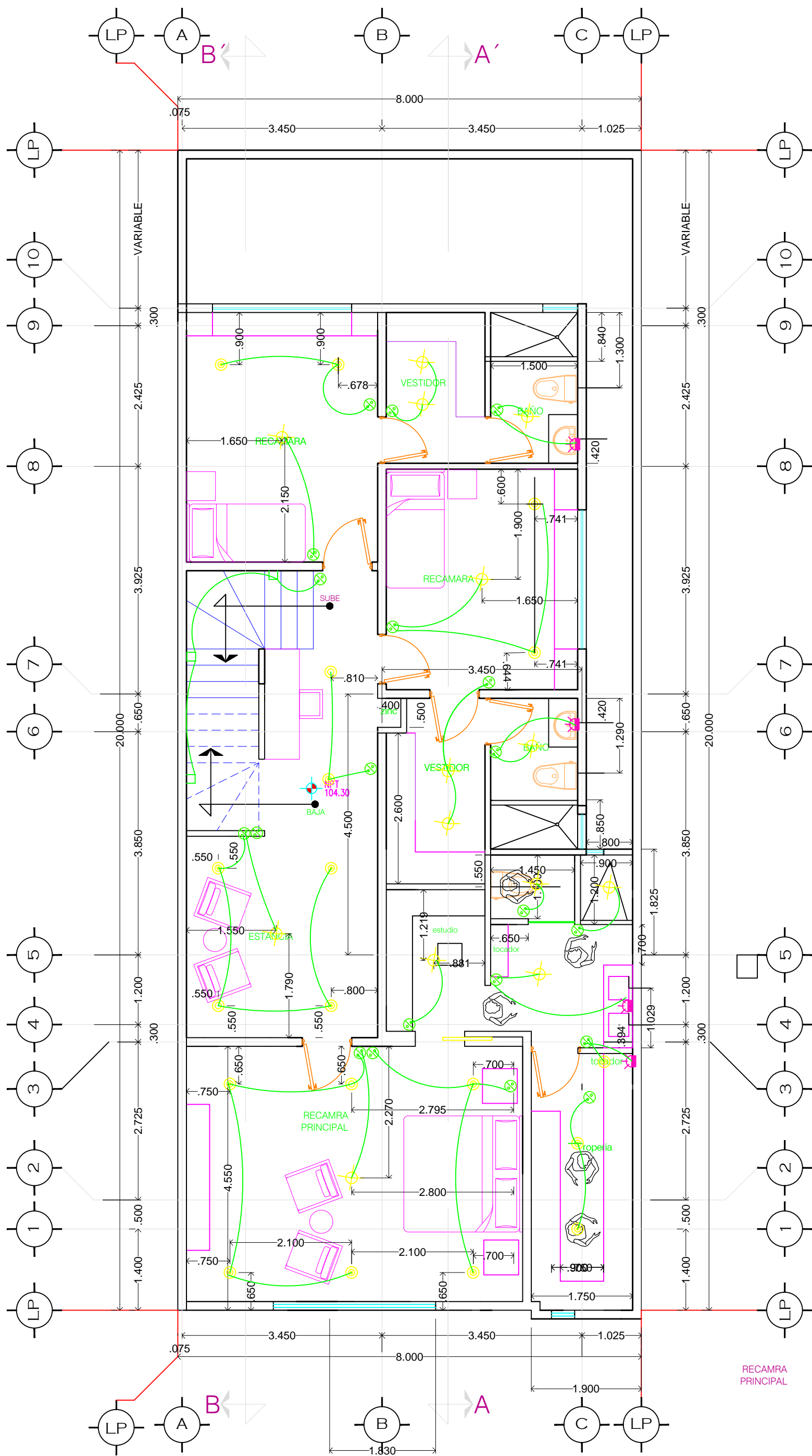
PLANTA ALTA casa tipo con terraza
